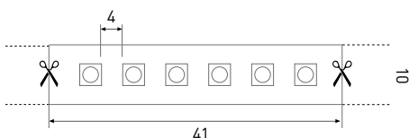
DISTANZA PUNTI DI TAGLIO E DISTANZA DIODI
